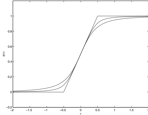
Figure 8: Função \phi_X – Efeito da Variação do Parâmetro \tau
