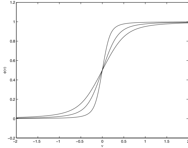
Figure 7: Função \phi_X — Efeito da Variação do Parâmetro \lambda
