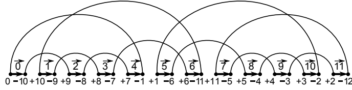
Figura 2.1: G([0 \ 10 \ 9 \ 8 \ 7 \ 1 \ 6 \ 11 \ 5 \ 4 \ 3 \ 2 \ 12]) . O conjunto de ciclos é \{C_1 = \langle 0 \ 2 \ 4 \rangle, C_2 = \langle 1 \ 3 \ 6 \rangle, C_3 = \langle 5 \ 8 \ 10 \rangle, C_4 = \langle 7 \ 9 \ 11 \rangle\} . Os ciclos C_2 e C_3 se intersectam, mas não se intercalam; os ciclos C_1 e C_2 se intercalam, e da mesma forma os ciclos C_3 e C_4 . O ciclo C_1 é o ciclo mais à esquerda.
