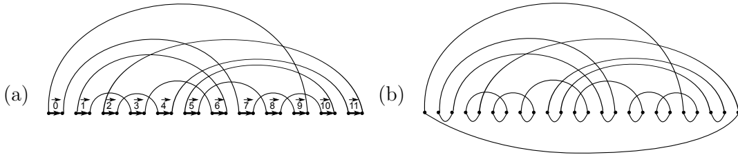
Figura 2.2: (a) Configuração completa F = \{\langle 0 \ 7 \ 9 \rangle, \langle 1 \ 3 \ 6 \rangle, \langle 2 \ 4 \ 11 \rangle, \langle 5 \ 8 \ 10 \rangle\} , que não corresponde a permutação. (b) Configuração complementar F , obtida pela troca das arestas de realidade pelas arestas -\pi_i \pi_i e 0 - \pi_{n+1} .
