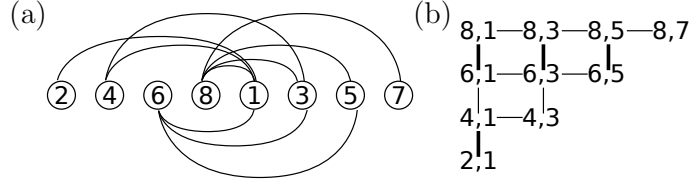
Figura 1.3: (a) PG([0\ 2\ 4\ 6\ 8\ 1\ 3\ 5\ 7\ 9]) (b) A_{[0\ 2\ 4\ 6\ 8\ 1\ 3\ 5\ 7\ 9]}^a .
